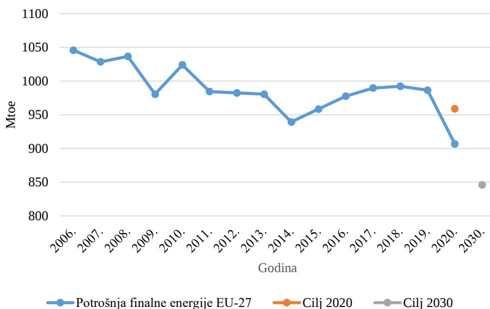
Slika 5 Potrošnja finalne energije – EU 27
